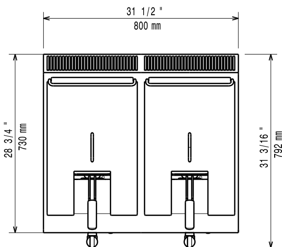
Boven aanzicht
